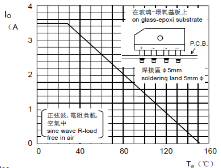
I o -T a 曲線 I o -T a Curve
